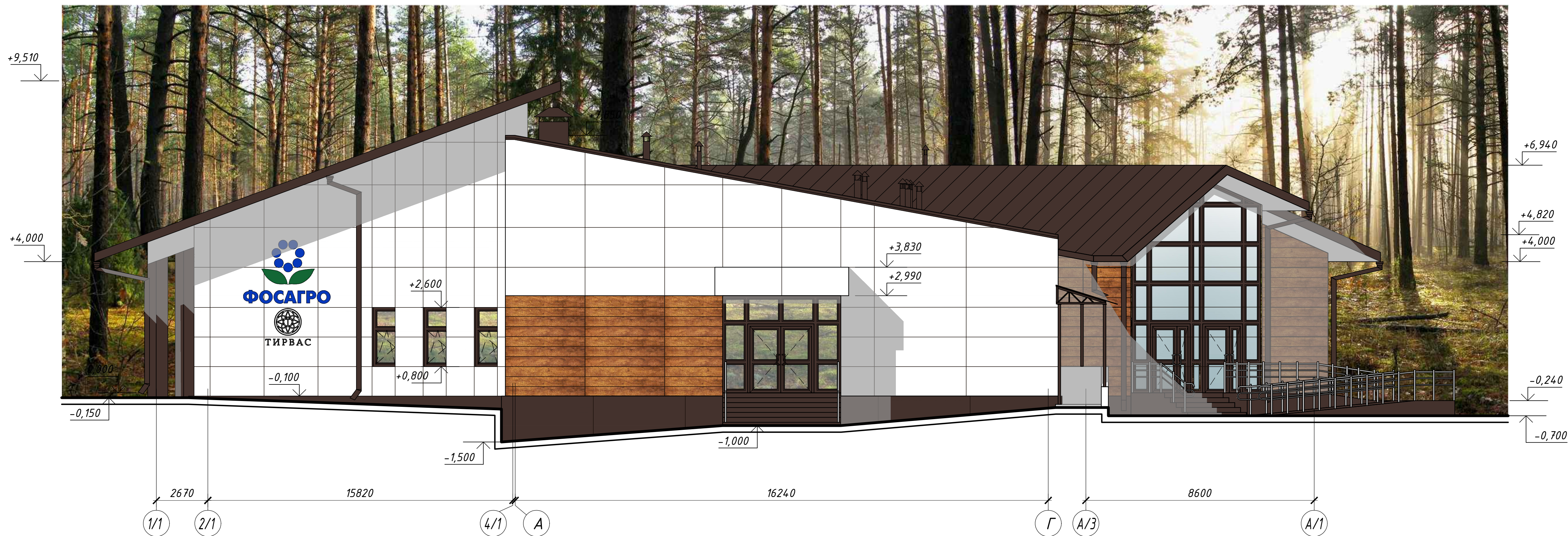
Фасад 1 /1 - А/1
