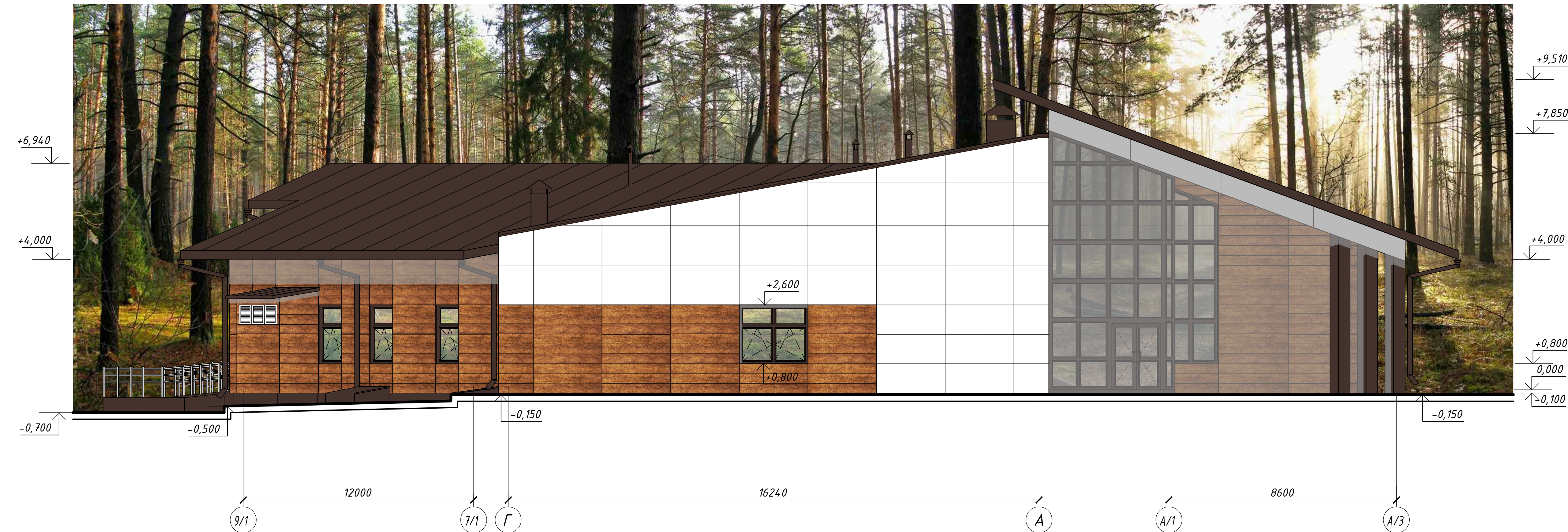
Фасад 9/1- А/3
