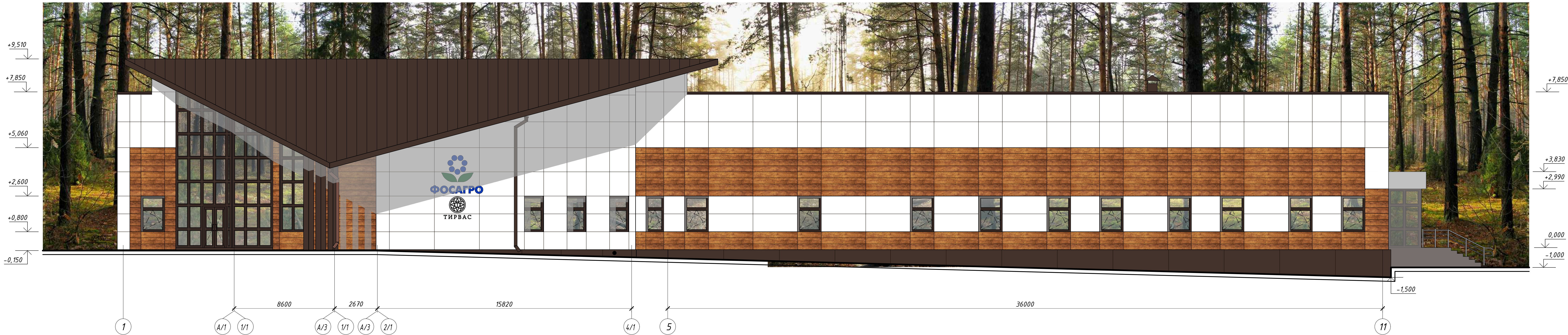
Фасад 1 - 11
